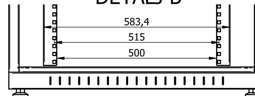
DETALJ B
