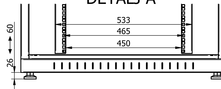
DETALJ A
